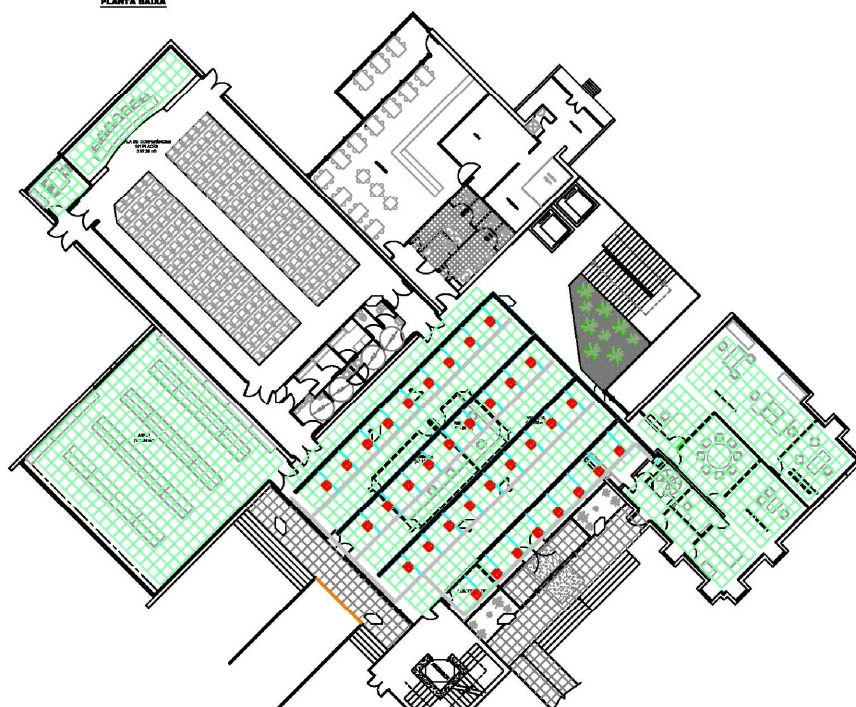
PLANTA BAJA
